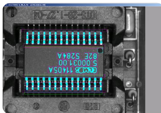
Bild 1: Kontrons KISS-Server werden von Asentics z.B. in einer Mikrochip-Prüfanlage mit Bauteilen für die Airbag-Steuerung in Autos eingesetzt. Die Prozessaufnahme eines Chips zeigt die relevanten Prüfbereiche der Bauteilkontrolle.
